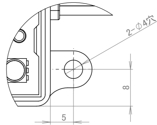
詳細図 A 2個所同形状
