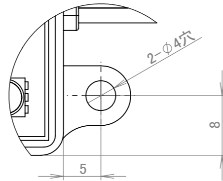
詳細図 A 2箇所同形状
